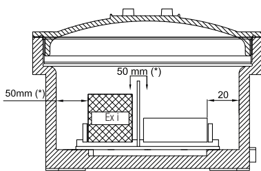
Esempio di unità d'interfaccia (con apparecchiature associate) completa di separatore
