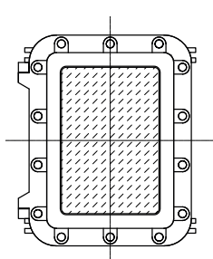
DETTAGLIO EJB-4/3020 EJB-4B/3020
