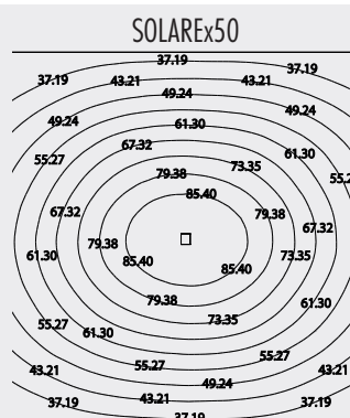
Illuminamento a pavimento riferito al sistema SOLAREx50 espresso in lux con armatura posta a h: 4m di altezza.
